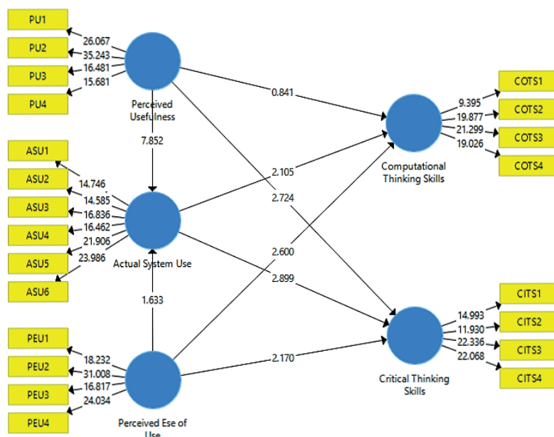
Figura 3. Resultado de T-statistic
