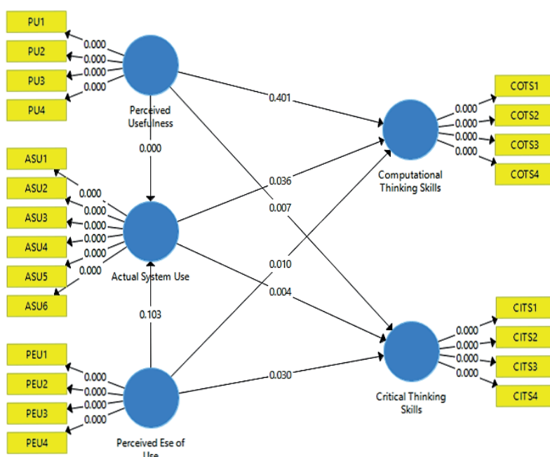
Figura 4. Resultado del P-value
